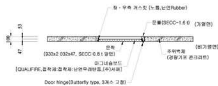
수평단면도
