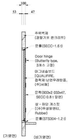
수직단면도
