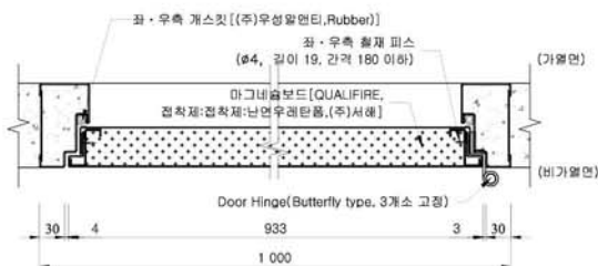
수평부분상세도
