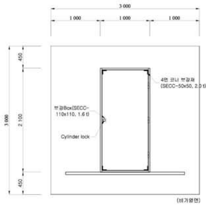
입면도
